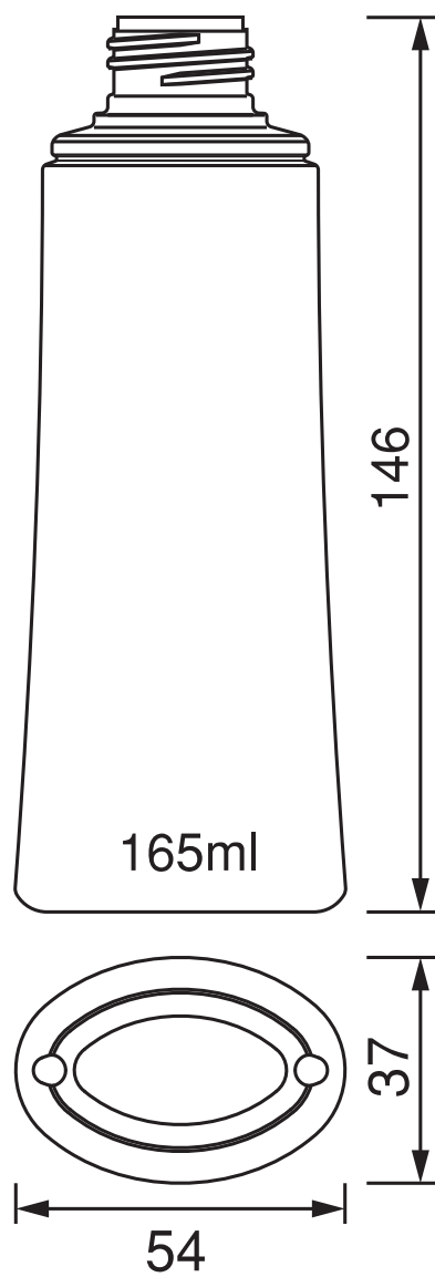
OC-150
