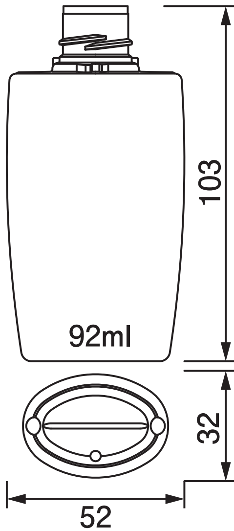
OHUV-80
