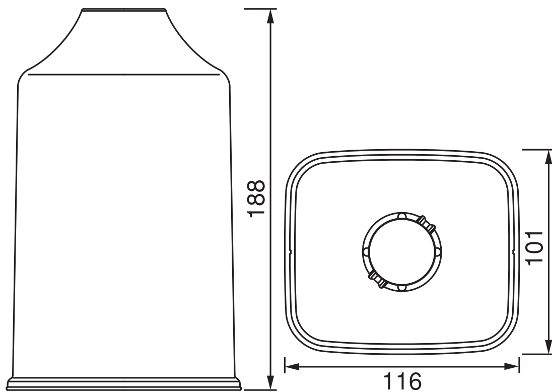
RPB-900・1000ケース RPB-900・1000Case
