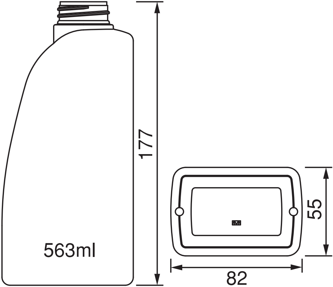
SPT-500
