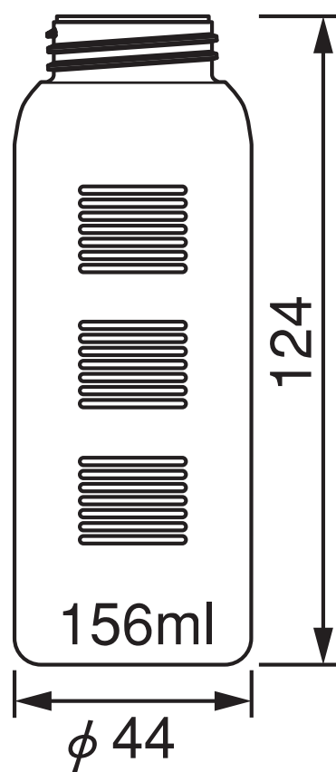
アプリケーションター120 Applicator 120
