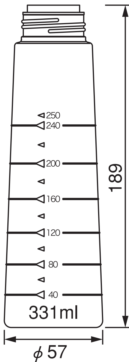
アプリケーターSS250 Applicator SS250
