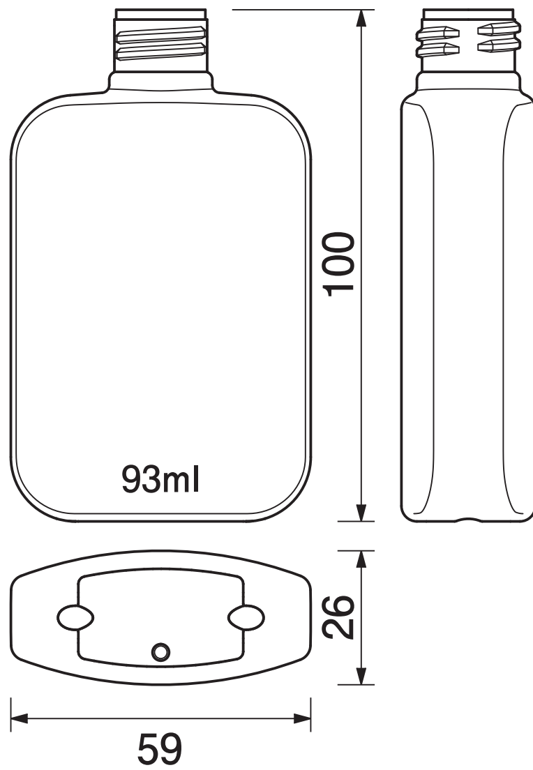
PPS-F80
