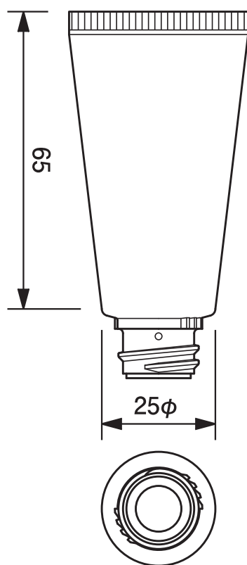
25φエアレスポンプチューブ -21.1 25mm dia. Airless Tube-21.1
