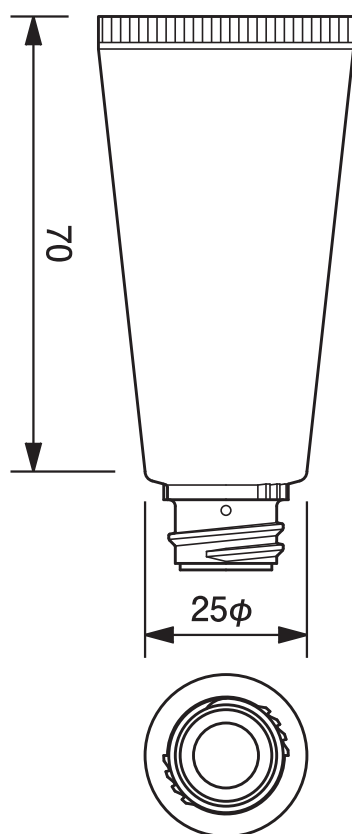
25φエアレスポンプチューブ -23.6 25mm dia. Airless Tube-23.6
