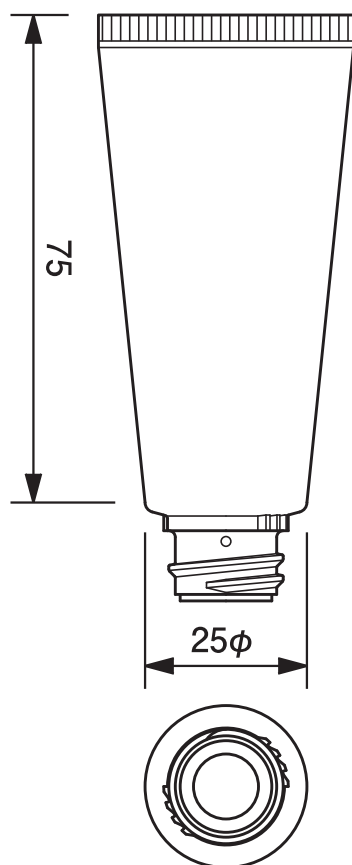
25φエアレスポンプチューブ -26.2 25mm dia. Airless Tube-26.2
