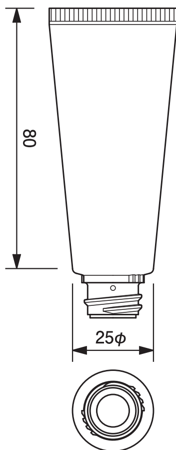
25φエアレスポンプチューブ -28.3 25mm dia. Airless Tube-28.3
