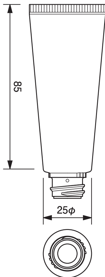
25φエアレスポンプチューブ -30.9 25mm dia. Airless Tube-30.9
