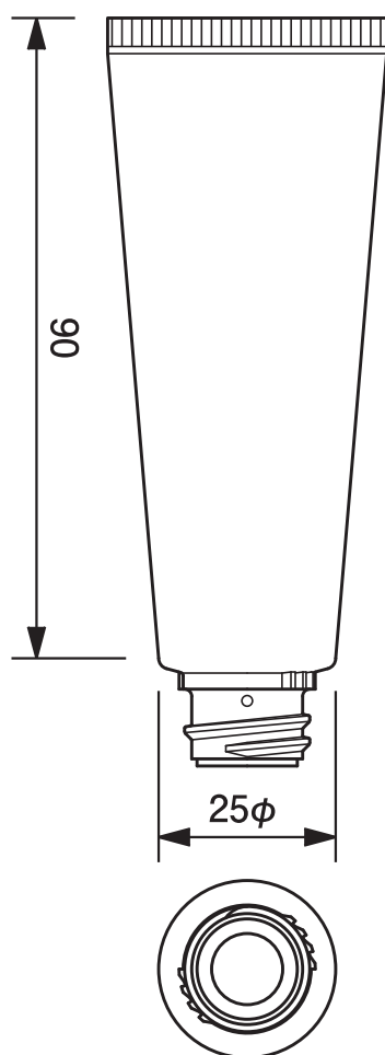
25φエアレスポンプチューブ -33.4 25mm dia. Airless Tube-33.4
