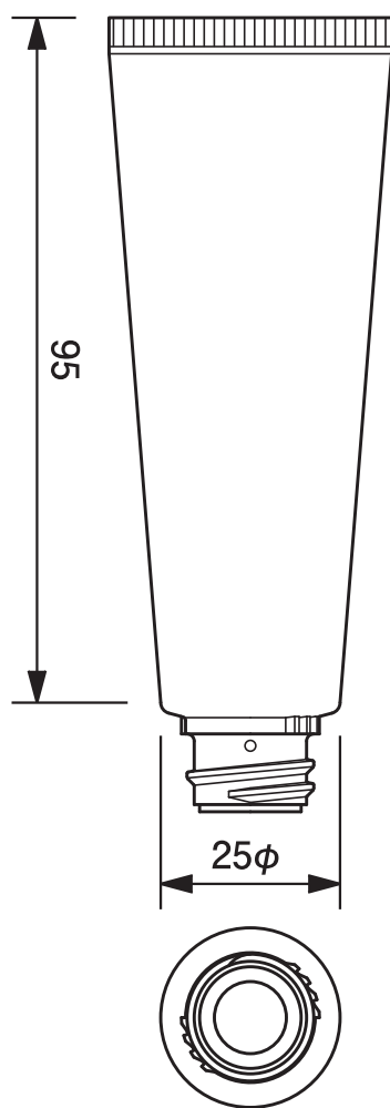
25φエアレスポンプチューブ -35.2 25mm dia. Airless Tube-35.2
