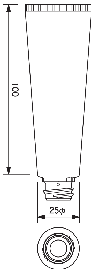
25φエアレスポンプチューブ -37.7 25mm dia. Airless Tube-37.7
