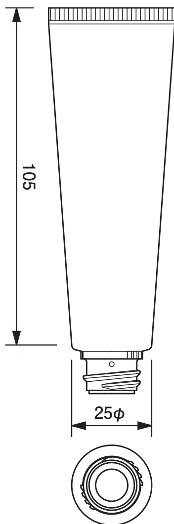
25φエアレスポンプチューブ -39.7 25mm dia. Airless Tube-39.7
