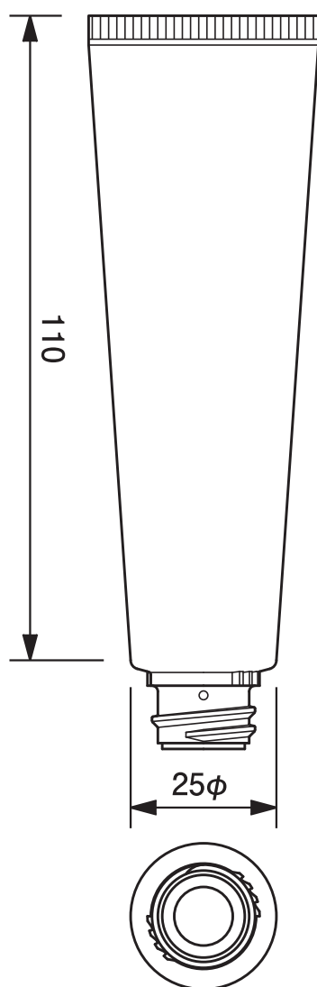
25φエアレスポンプチューブ -43 25mm dia. Airless Tube-43
