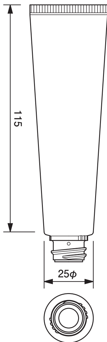
25φエアレスポンプチューブ -45.4 25mm dia. Airless Tube-45.4
