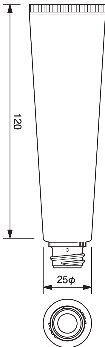
25φエアレスポンプチューブ -47.2 25mm dia. Airless Tube-47.2
