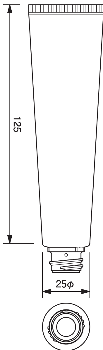
25φエアレスポンプチューブ -49.8 25mm dia. Airless Tube-49.8
