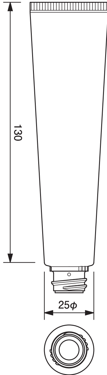
25φエアレスポンプチューブ -52.2 25mm dia. Airless Tube-52.2
