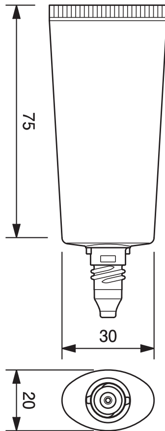
25φオーバルチューブ -24.8 25mm dia. Oval Tube-24.8
