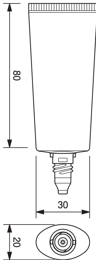
25φオーバルチューブ -27.5 25mm dia. Oval Tube-27.5
