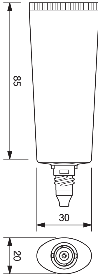
25φオーバルチューブ -29.9 25mm dia. Oval Tube-29.9
