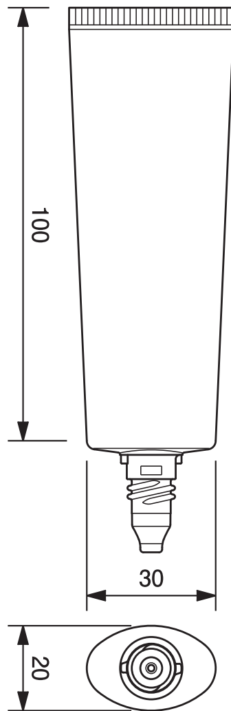
25φオーバルチューブ -37.2 25mm dia. Oval Tube-37.2
