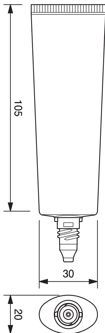
25φオーバルチューブ -39.1 25mm dia. Oval Tube-39.1
