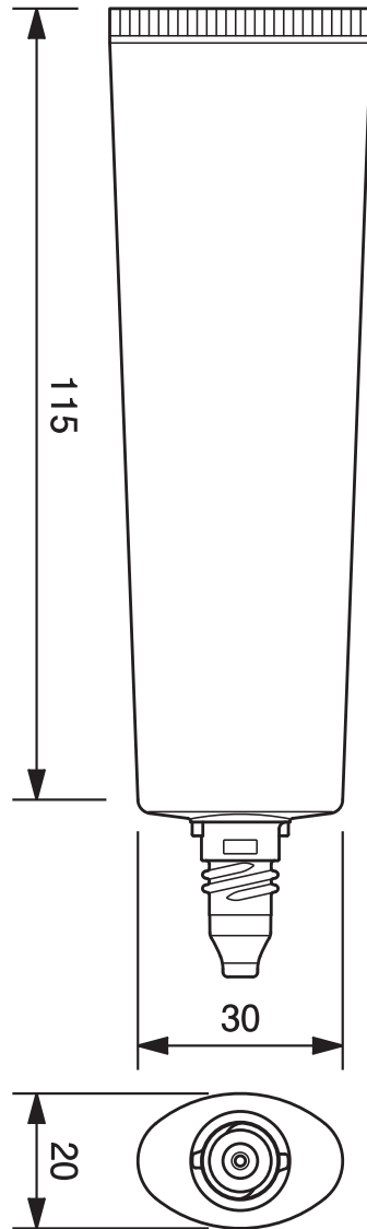
25φオーバルチューブ -44 25mm dia. Oval Tube-44
