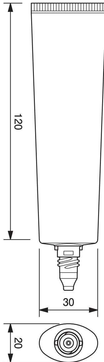
25φオーバルチューブ -46 25mm dia. Oval Tube-46
