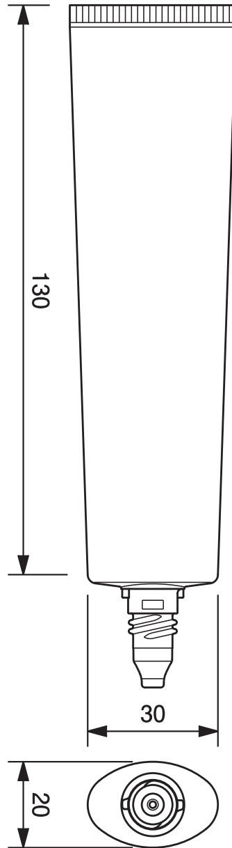
25φオーバルチューブ -51.3 25mm dia. Oval Tube-51.3
