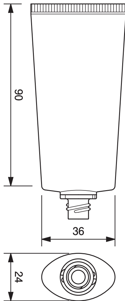
TN-30φオーバルチューブ -42.7 TN-30mm dia. Oval Tube-42.7
