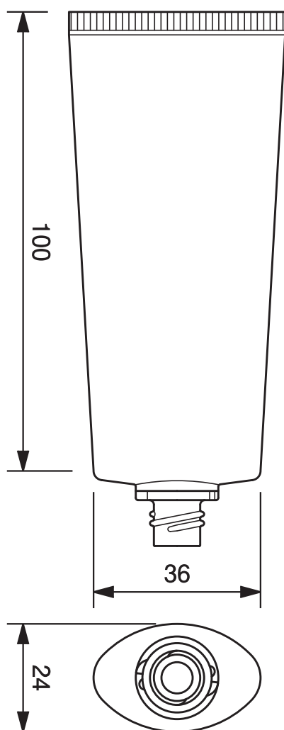
TN-30φオーバルチューブ -49.5 TN-30mm dia. Oval Tube-49.5
