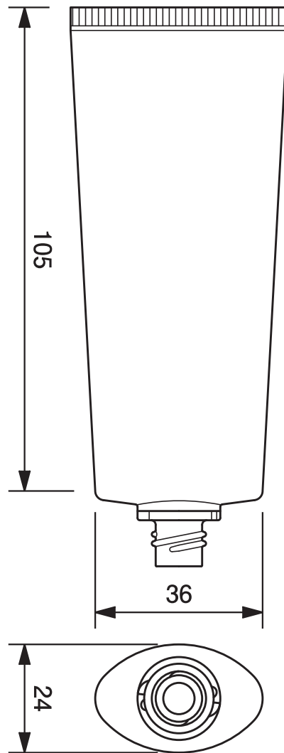
TN-30φオーバルチューブ -53.1 TN-30mm dia. Oval Tube-53.1
