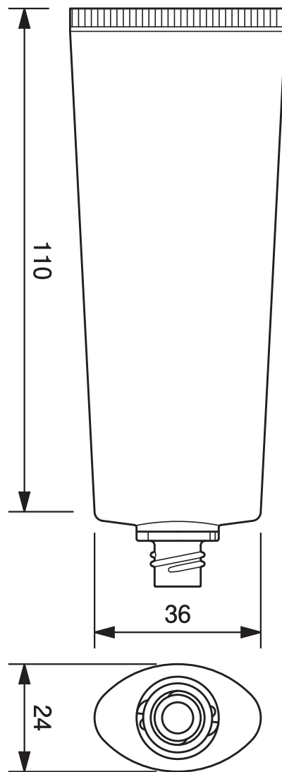
TN-30φオーバルチューブ -57.3 TN-30mm dia. Oval Tube-57.3
