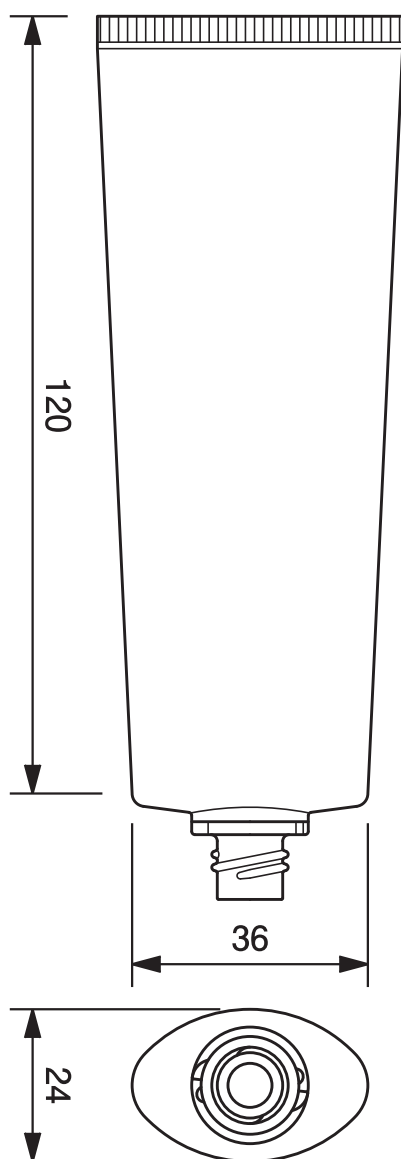
TN-30φオーバルチューブ -63.0 TN-30mm dia. Oval Tube-63.0
