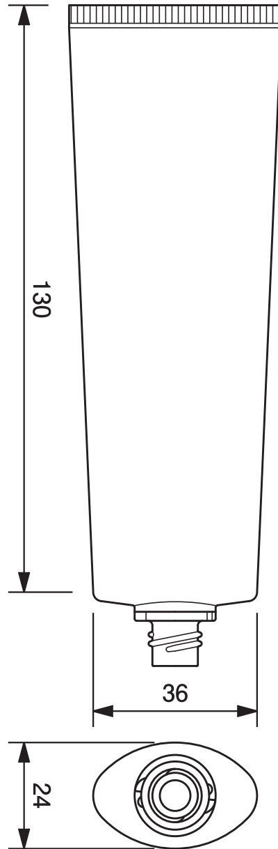
TN-30φオーバルチューブ -70.7 TN-30mm dia. Oval Tube-70.7
