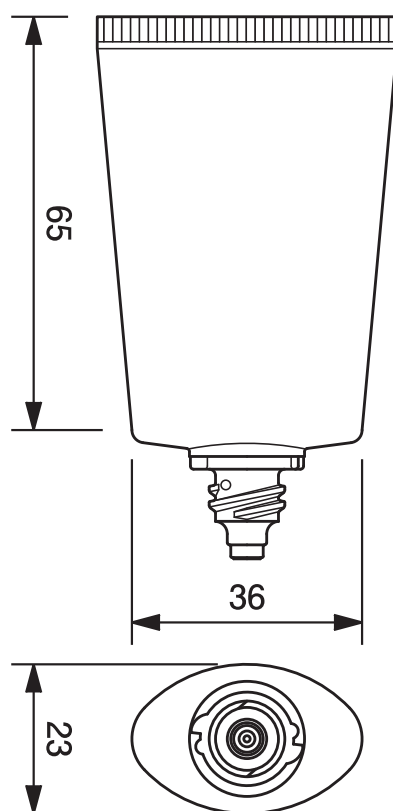
30φオーバルチューブ -27.1 30mm dia. Oval Tube-27.1
