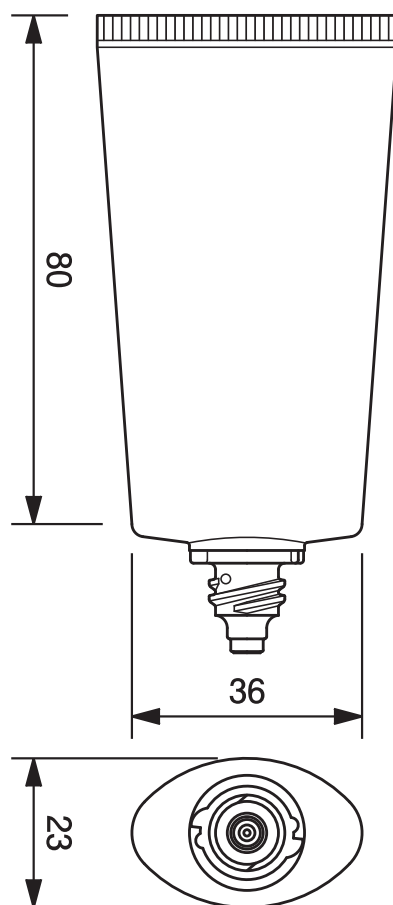
30φオーバルチューブ -35.8 30mm dia. Oval Tube-35.8
