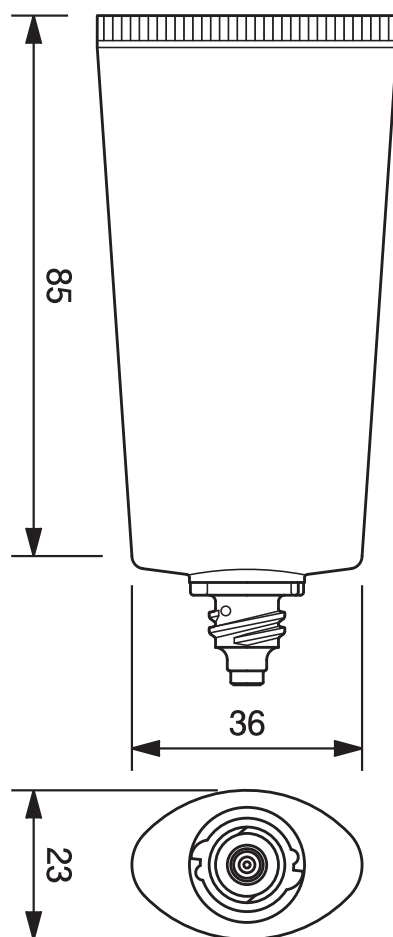
30φオーバルチューブ -39.7 30mm dia. Oval Tube-39.7
