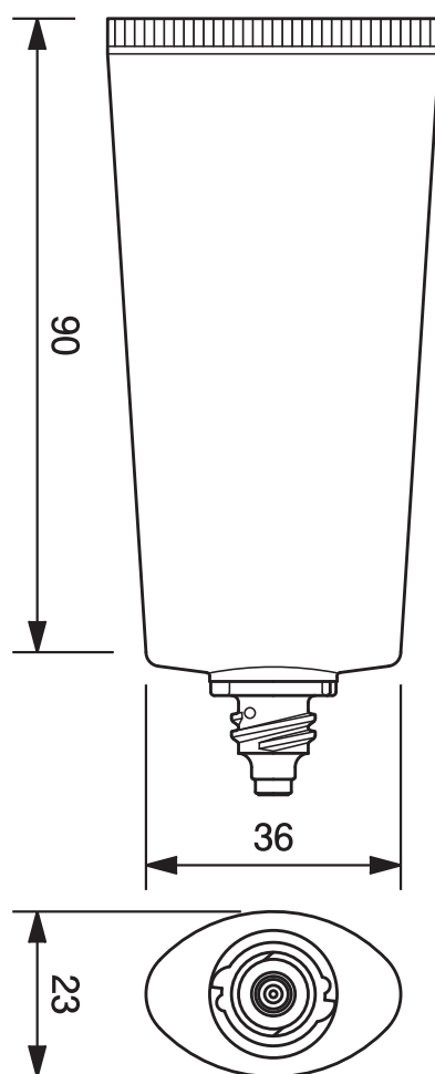
30φオーバルチューブ -42.7 30mm dia. Oval Tube-42.7
