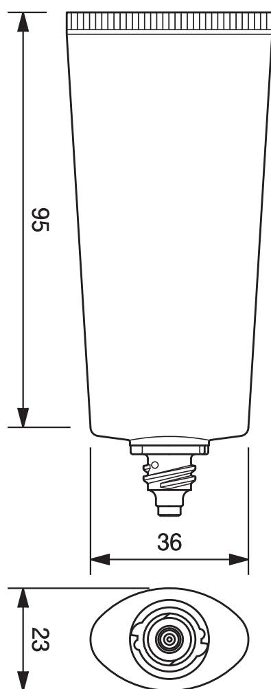
30φオーバルチューブ -46.2 30mm dia. Oval Tube-46.2
