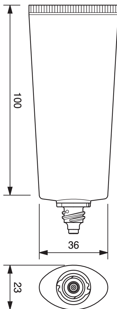
30φオーバルチューブ -49.5 30mm dia. Oval Tube-49.5
