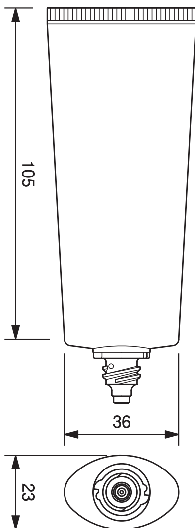
30φオーバルチューブ -53.1 30mm dia. Oval Tube-53.1
