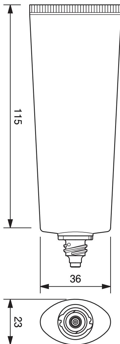
30φオーバルチューブ -60.0 30mm dia. Oval Tube-60.0
