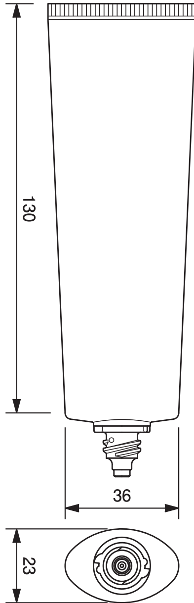
30φオーバルチューブ -70.7 30mm dia. Oval Tube-70.7
