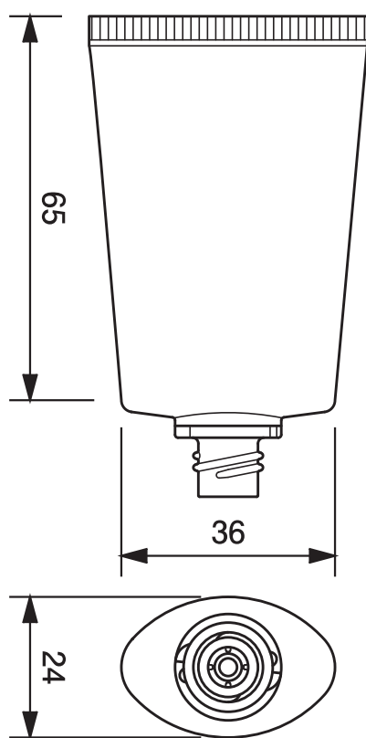
TV-30φオーバルチューブ -27.1 TV-30mm dia. Oval Tube-27.1
