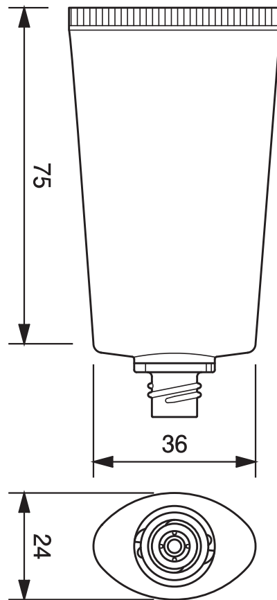
TV-30φオーバルチューブ -33.6 TV-30mm dia. Oval Tube-33.6
