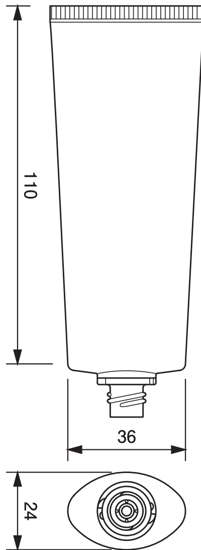
TV-30φオーバルチューブ -57.3 TV-30mm dia. Oval Tube-57.3
