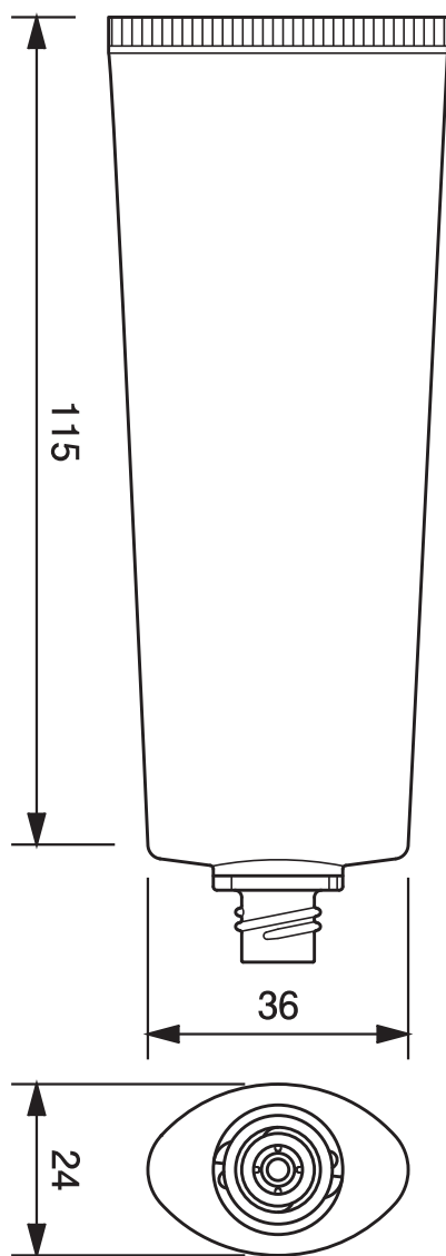
TV-30φオーバルチューブ -60.0 TV-30mm dia. Oval Tube-60.0
