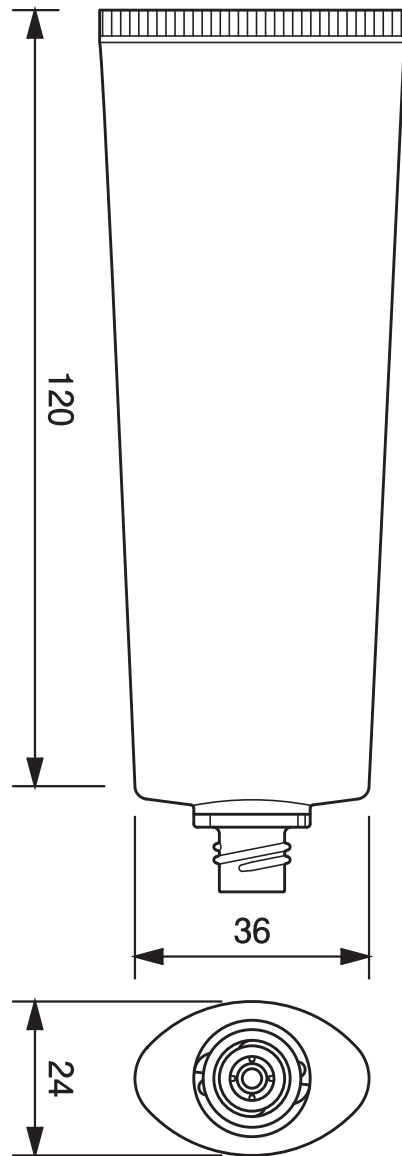
TV-30φオーバルチューブ -63.0 TV-30mm dia. Oval Tube-63.0
