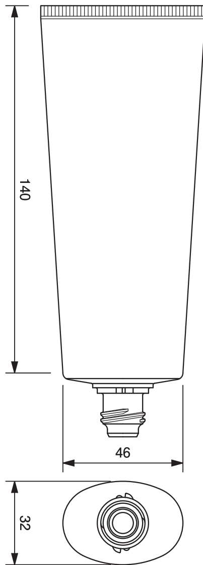
40φオーバルチューブ -134.5 40mm dia. Oval Tube-134.5
